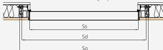
DVEŘE HARMONI INVEST (OTEVÍRÁNÍ VEN) ODZ
