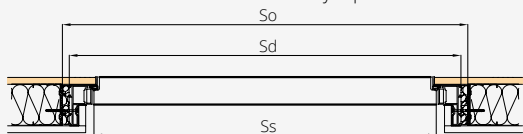
DVEŘE HARMONY INVEST PRO otvírání dovnitř s obložkovým panelem
