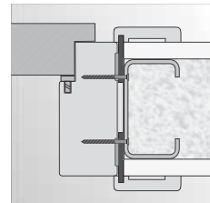
montáž na vruty do stěny ze sádkrotonu
