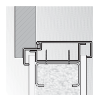
rohová zárubeň velká montáž na sádkrotonovou stěnu
