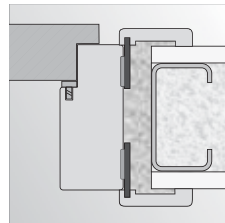
montáž na pěnu do stěny ze sádkrotonu
