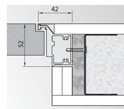
Reverzní podrážka (otevírané dovnitř)
