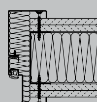
Rohová a doplnková zárubňa Montáž skrutkovaním
