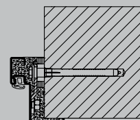
Rohová zárubňa so skrytou montážou pomocou hmoždiniek
