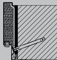
Obvodová zárubňa Diagonálne upevnenie do MW 175
